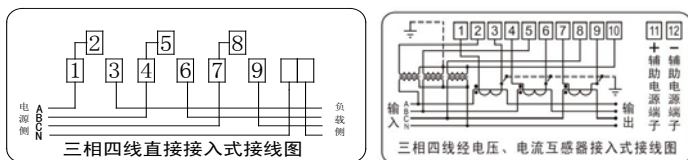
图 2: 主端子接线图
