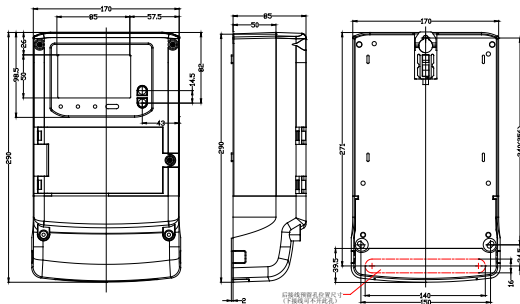
图 1: 安装尺寸图
