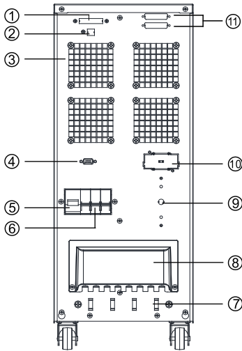
3C15KS/3C20KS
