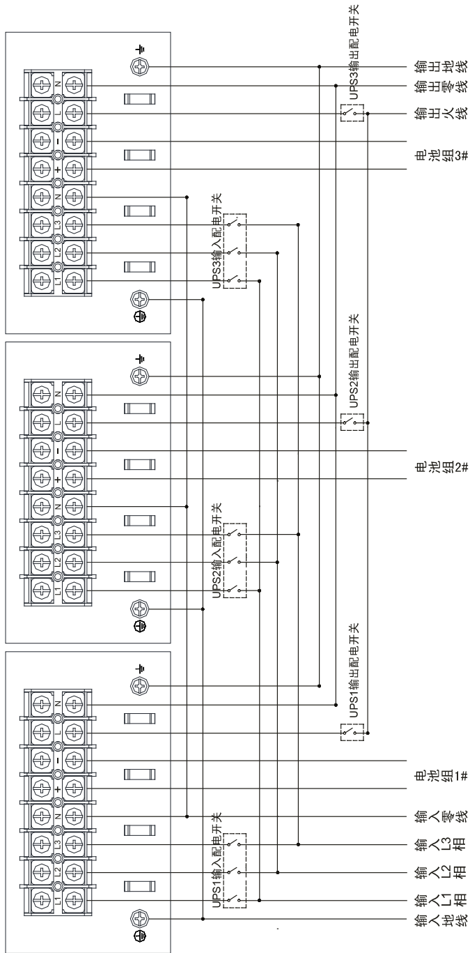
3C15KS/3C20KS 并机接线图
